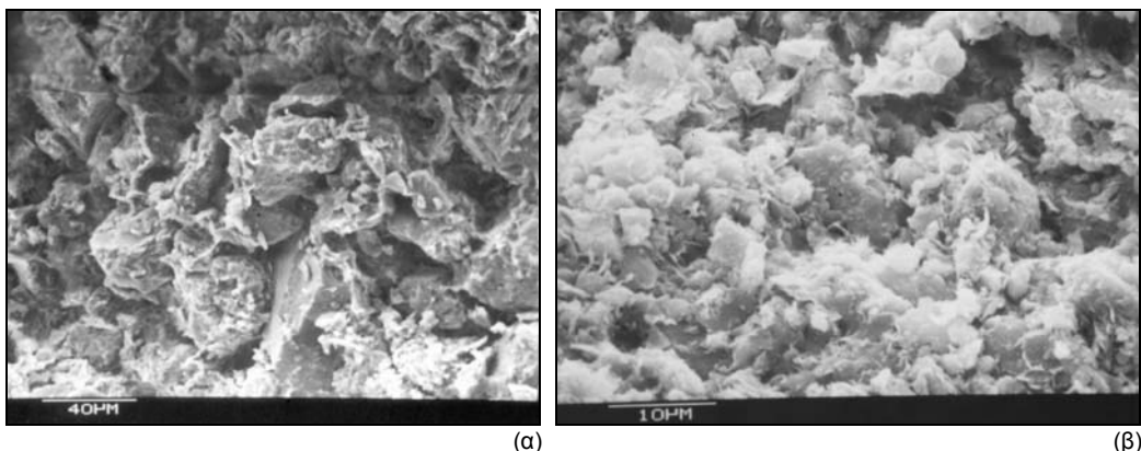
Σχήμα 4. Μικροφωτογραφίες SEM που δείχνουν τη μικροδομή των δειγμάτων 5 (α) (x500) και 21 (β) (x2000).
