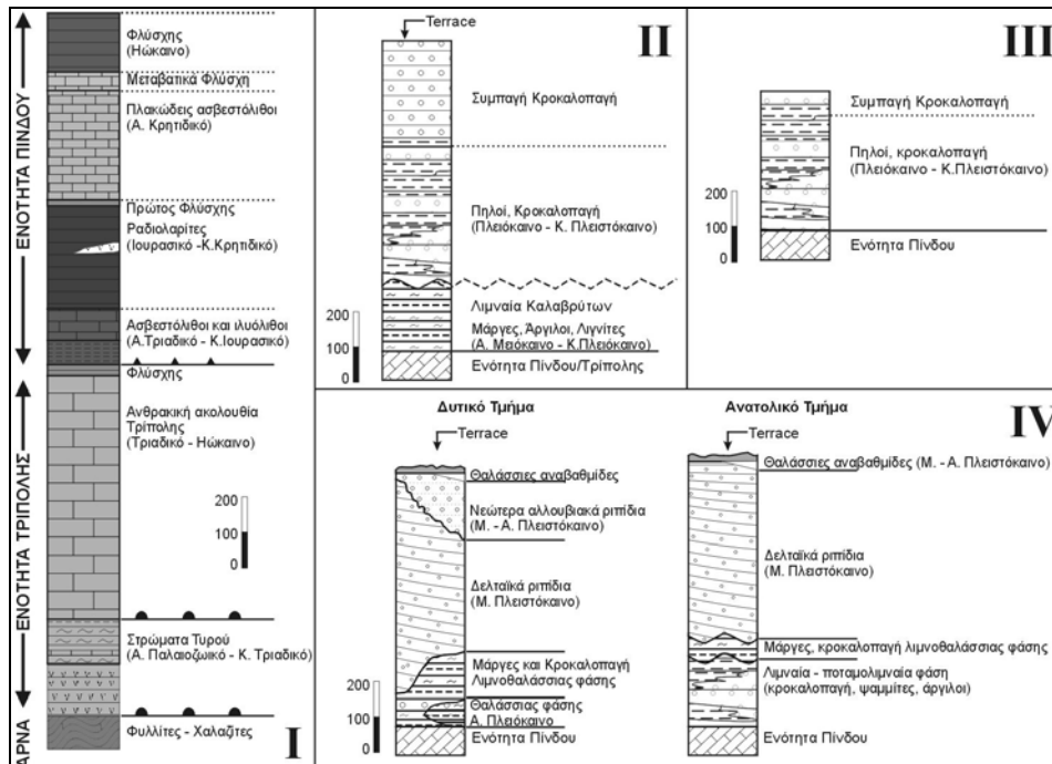
Εικ. 2. Απλοποιημένες στήλες του φύλλου ΑΙΓΙΟ, των αλπικών σχηματισμών (I) και των μεταλπικών της λεκάνης Καλαβρύτων (II), Βάλτας (III) και της παραλιακής λεκάνης (IV).
