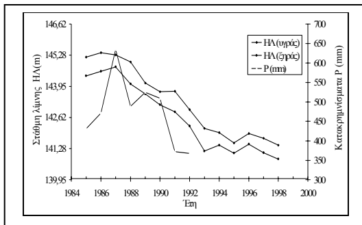
Σχήμα 4. Διάγραμμα στάθμης λίμνης – χρόνου και μεταβολής στάθμης λίμνης (ΔΗ L )-χρόνου (t)
