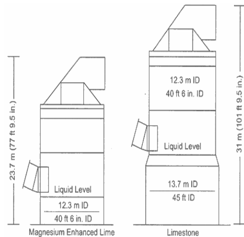
Σχήμα 2. Διαστάσεις των πύργων καθαρισμού που χρησιμοποιούν άσβεστο και ασβεστόλιθο σε μια μονάδα παραγωγής ενέργειας. Πηγή: (Nolan, 2000).
