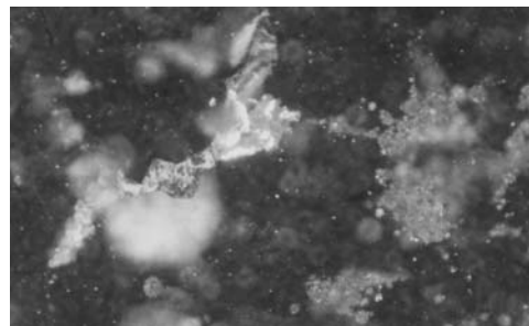
Σχήμα 11. Φυλλάρια χρυσού στο Πέραμα (<10μ.). Μικροφωτογραφία X 320, + N, και λάδι.
