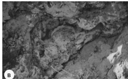
Σχήμα 3. Χαλαζιακή φλέβα στο Πέραμα. SiO 2 με κolloειδείς και φλοιώδεις μορφές.
