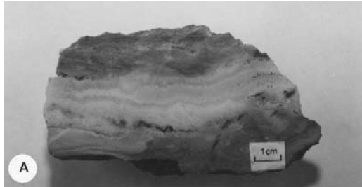
Σχήμα 6. Κολλοειδείς και ζωνώδεις μορφές χαλαζία στο Πέραμα.
