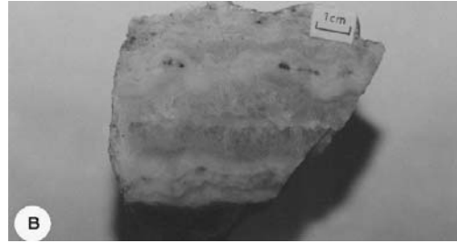
Σχήμα 7. Κτενοειδής και ζωνώδης χαλαζίας στο Πέραμα.
