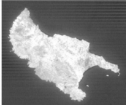
Σχ. 5. Εικόνα δείκτη βλάστησης NDVI της Νήσου Ζακύνθου
